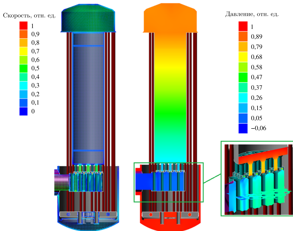
Рис. 5. Результаты теплогидравлического расчета реактора в программном комплексе FlowVision
