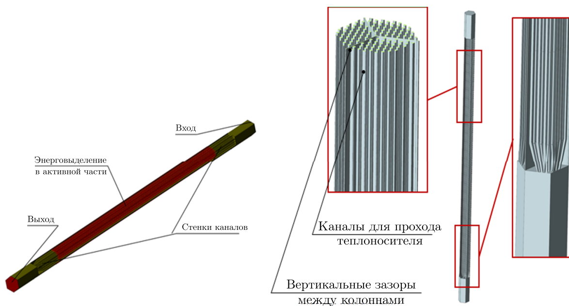
Рис. 2. Модель фрагмента графитовой кладки для расчета по FlowVision
