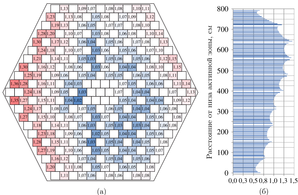
Рис. 4. Коэффициенты неравномерности энерговыделения по радиусу (а) и высоте (б) активной зоны
