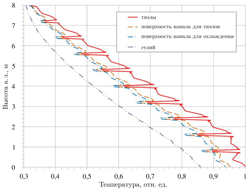
Рис. 7. Зависимость температуры колонны ТВС по высоте
