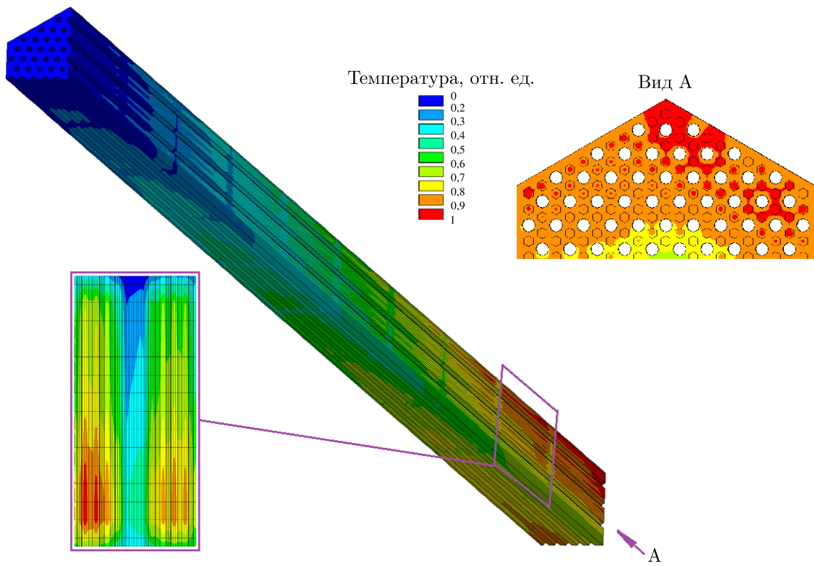
Рис. 6. Результаты расчета температурного состояния колонны ТВС
