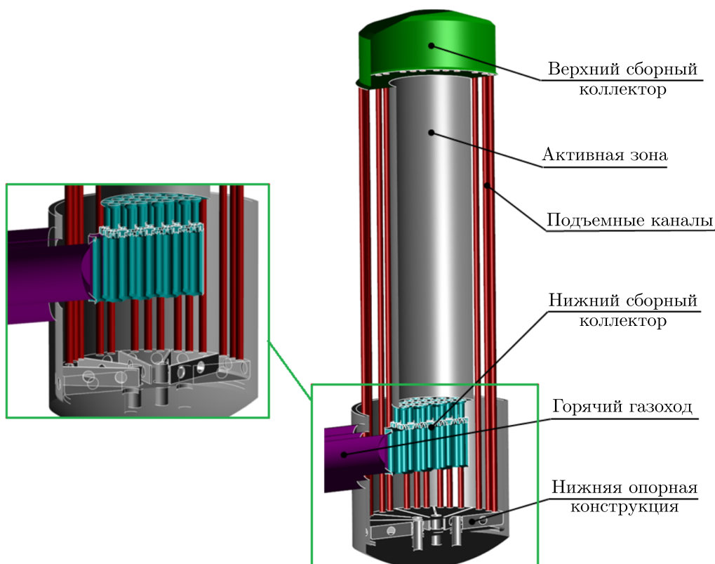
Рис. 1. Модель реактора для расчета по FlowVision
