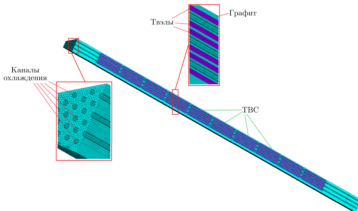
Рис. 3. Модель колонны ТВС (в разрезе)
