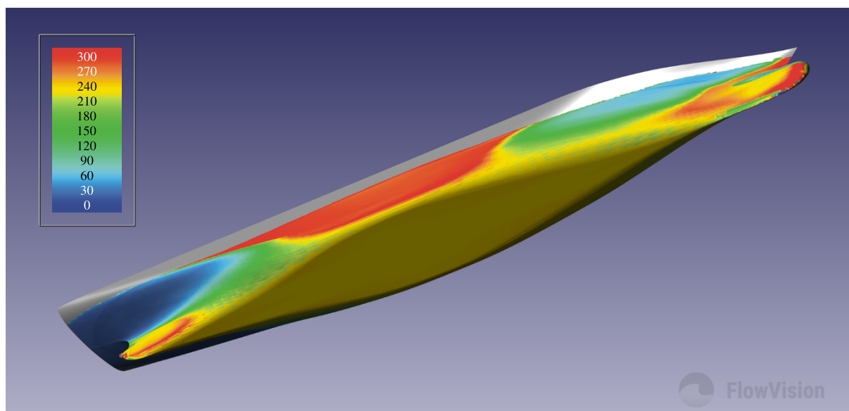
Рис. 3. Распределение y^+ по поверхности натурального корпуса KCS при скорости 24 узла ( Fr = 0,26 ), по сравнению с рис. 1 добавлена приповерхностная сетка с 186 тыс. расчетных ячеек
